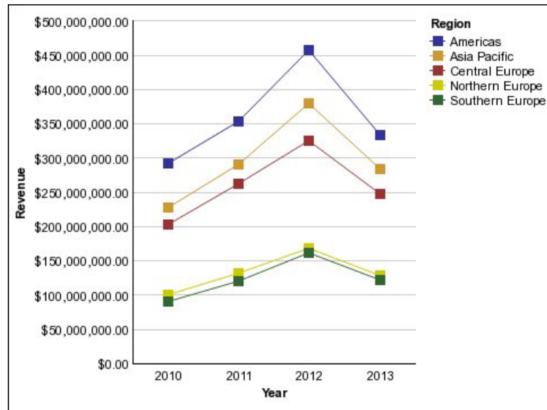
Рисунок 10. Пример линейной диаграммы
