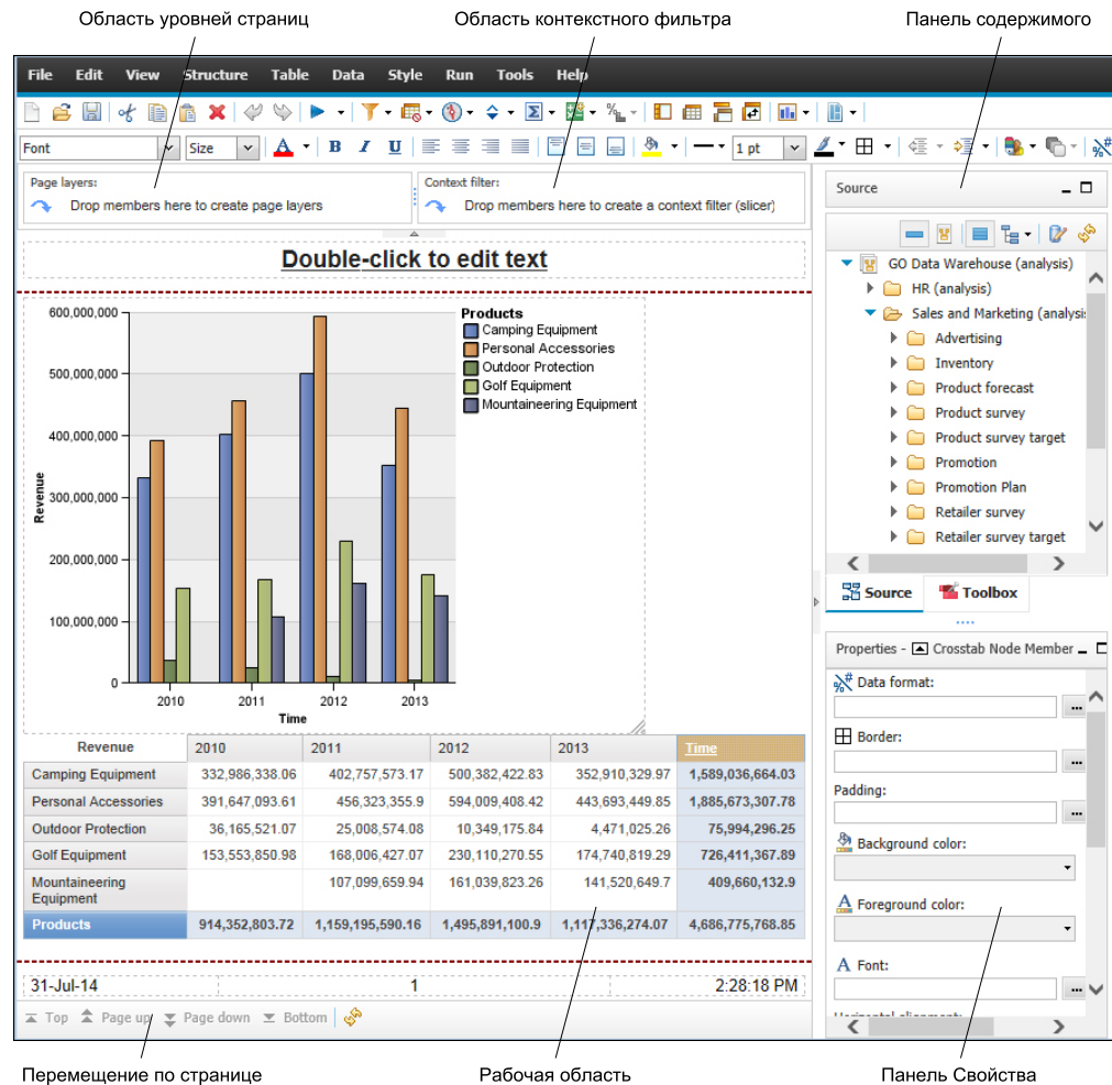
Рисунок 2. Пользовательский интерфейс Cognos Workspace Advanced
