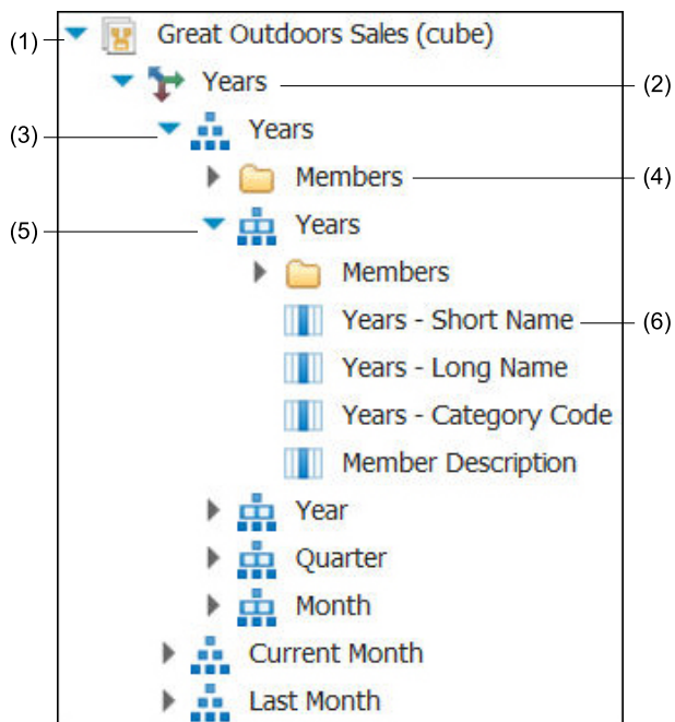
Рисунок 41. Дерево только многомерных данных
