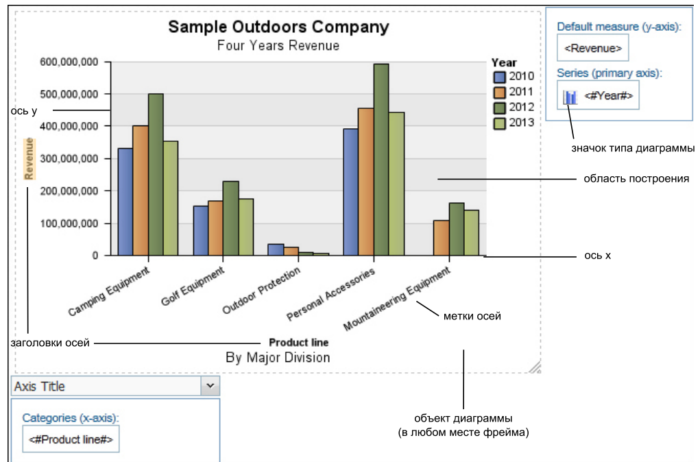
Рисунок 8. Столбчатая диаграмма с возможностями изменения с отмеченными элементами в Cognos Workspace Advanced
