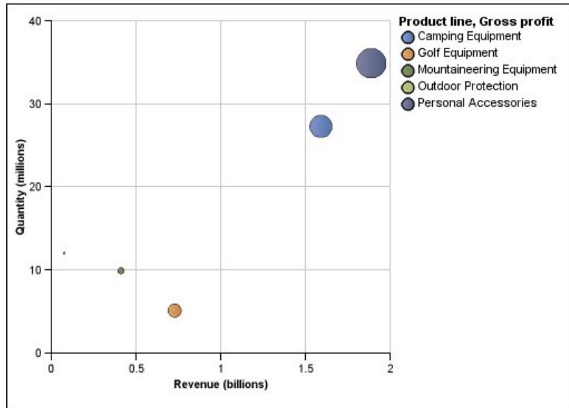
Рисунок 17. Пример пузырьковой диаграммы
