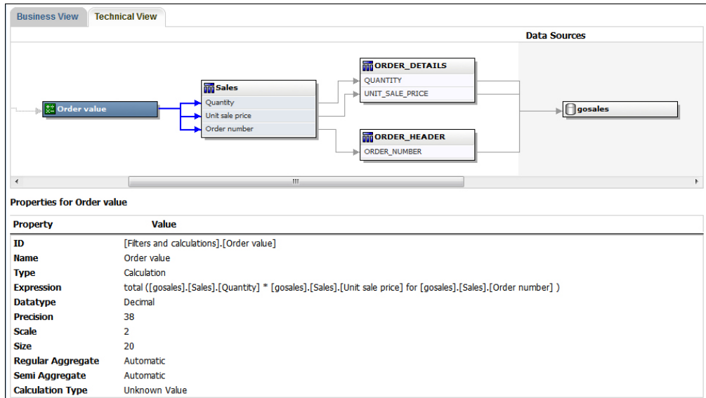
Рисунок 4. Техническое представление в средстве просмотра информации о происхождении IBM Cognos Business Intelligence
